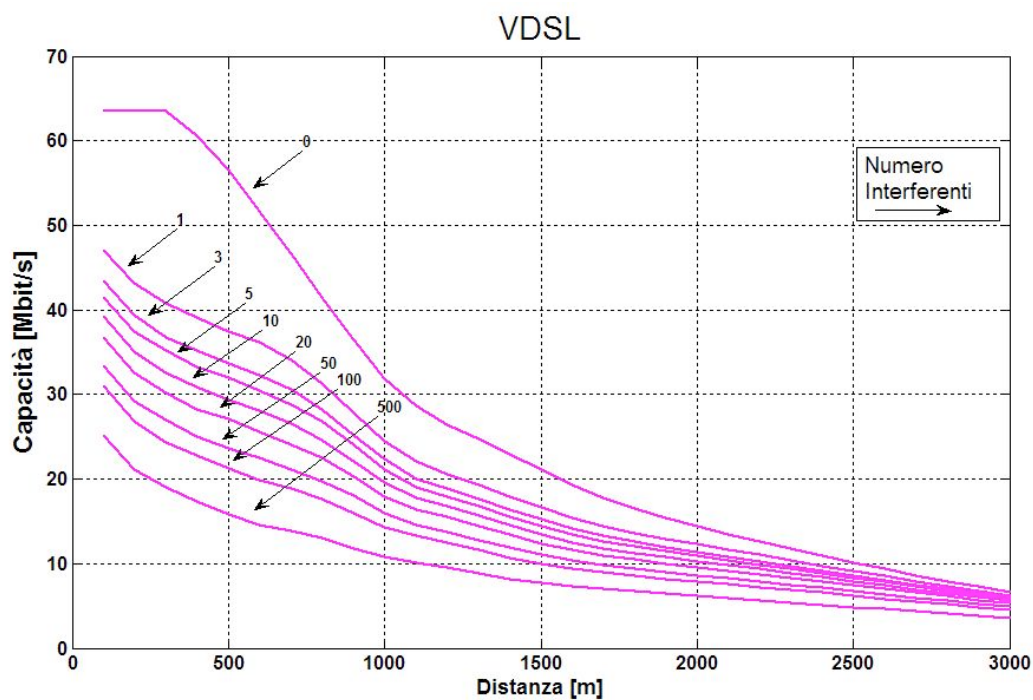
Figura 5 Downstream di un sistema VDSL
