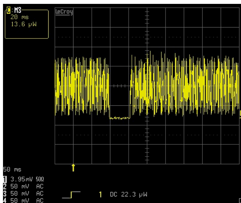
Figura 4 - 20 ms di interruzione
