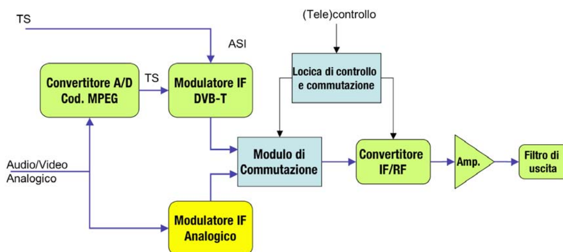
Figura 4.2: Schema di un trasmettitore dual-mode analogico/digitale
